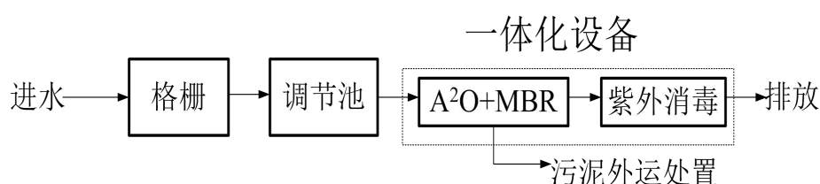
图2-3 污水处理工艺流程图
