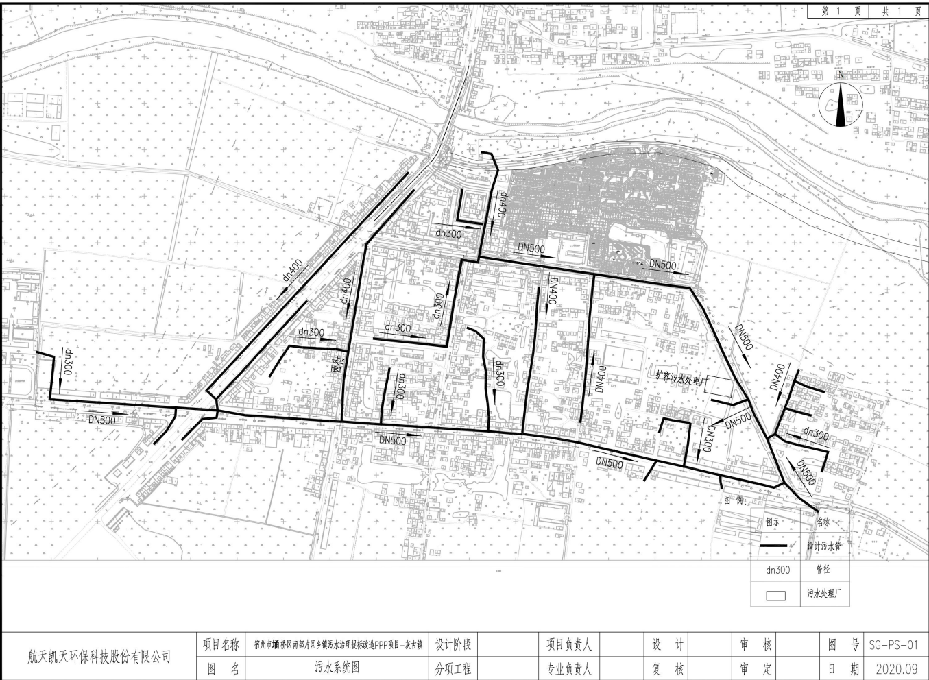
附图4 管网施工设计图
