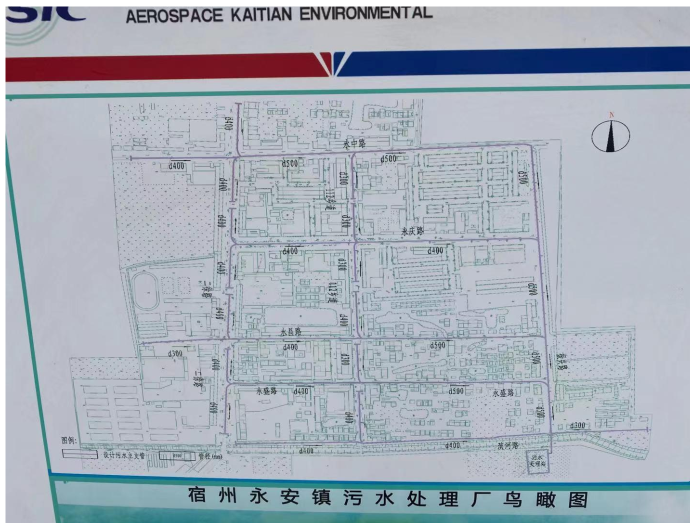
附图三 永安镇污水处理厂污水收集管网分布图
