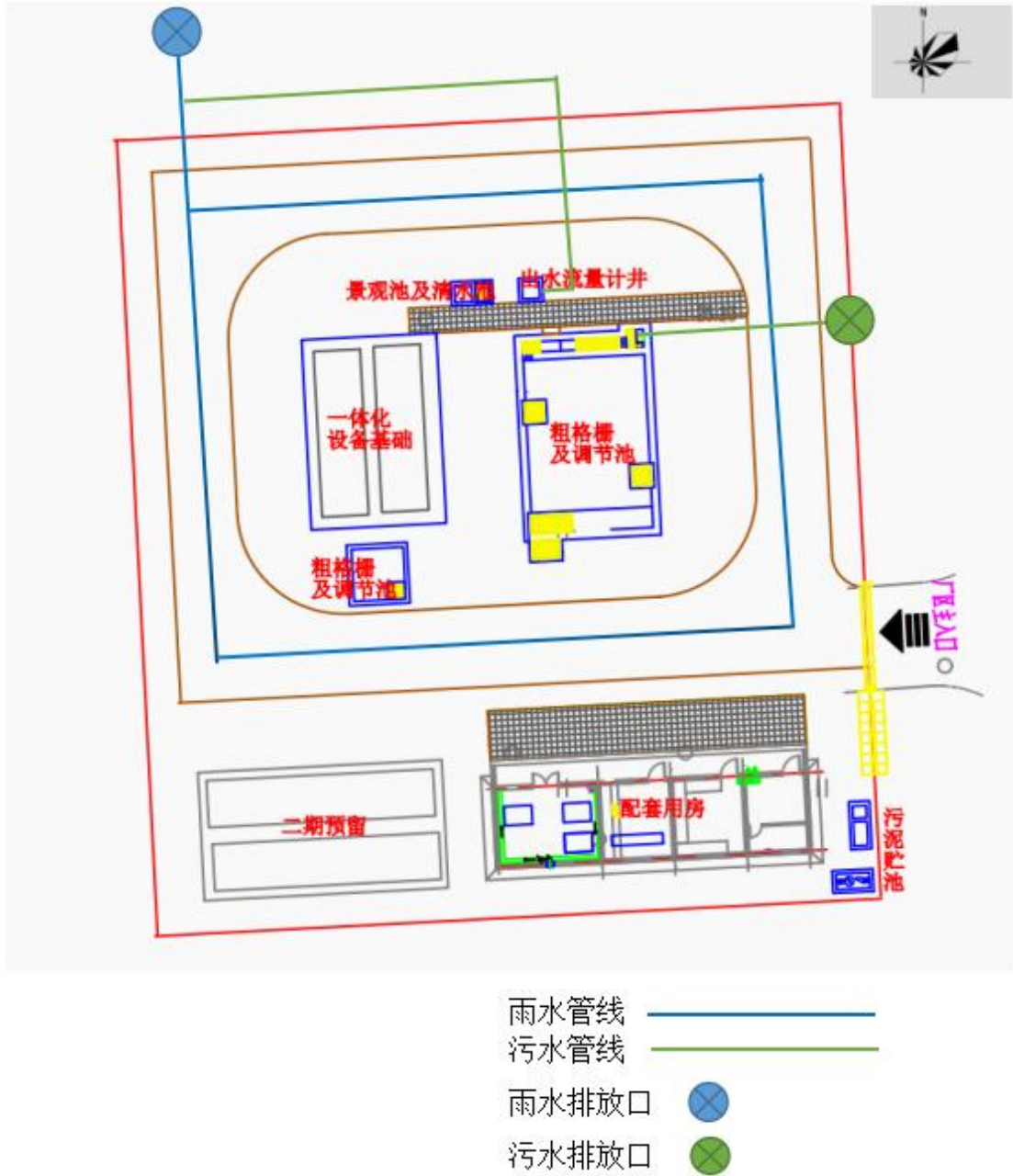
附图二 项目平面布置图及雨污管网图
