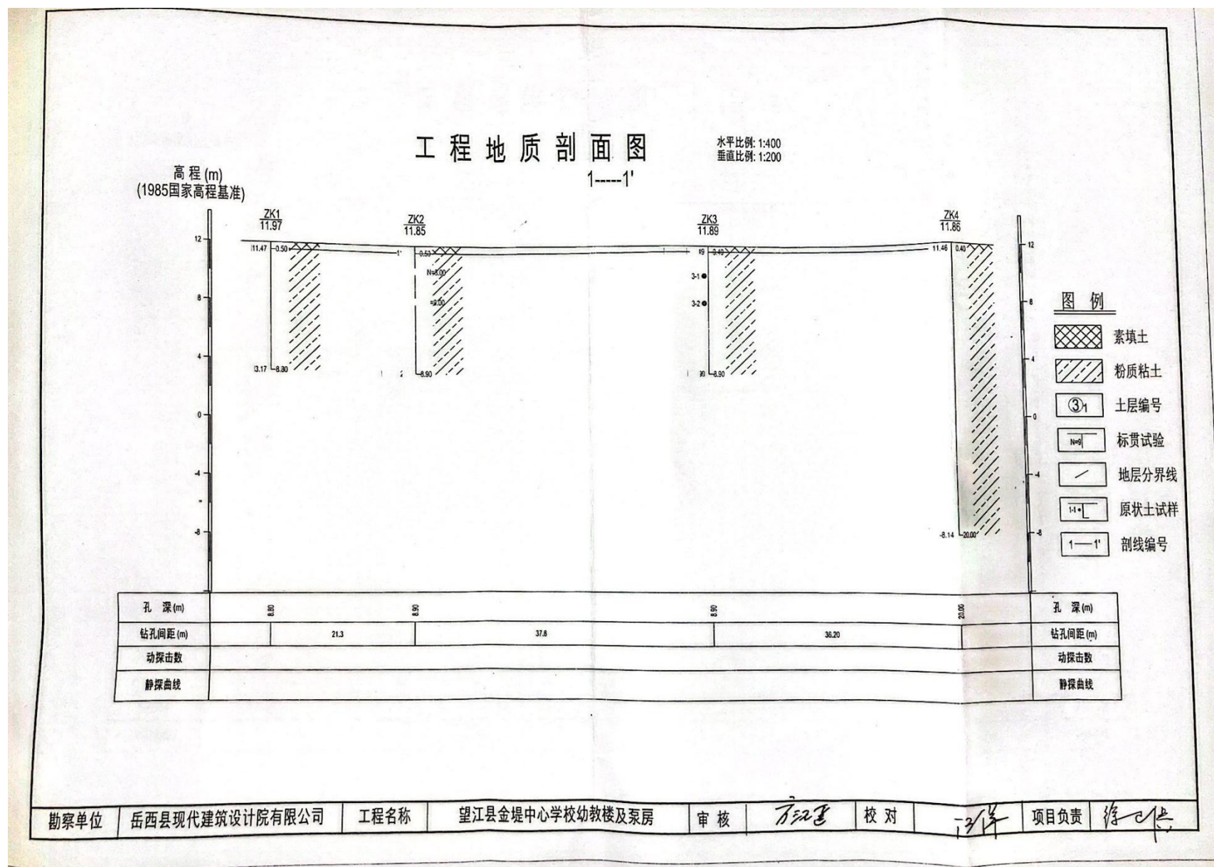
图 3-2 1-1'工程地质剖面图
