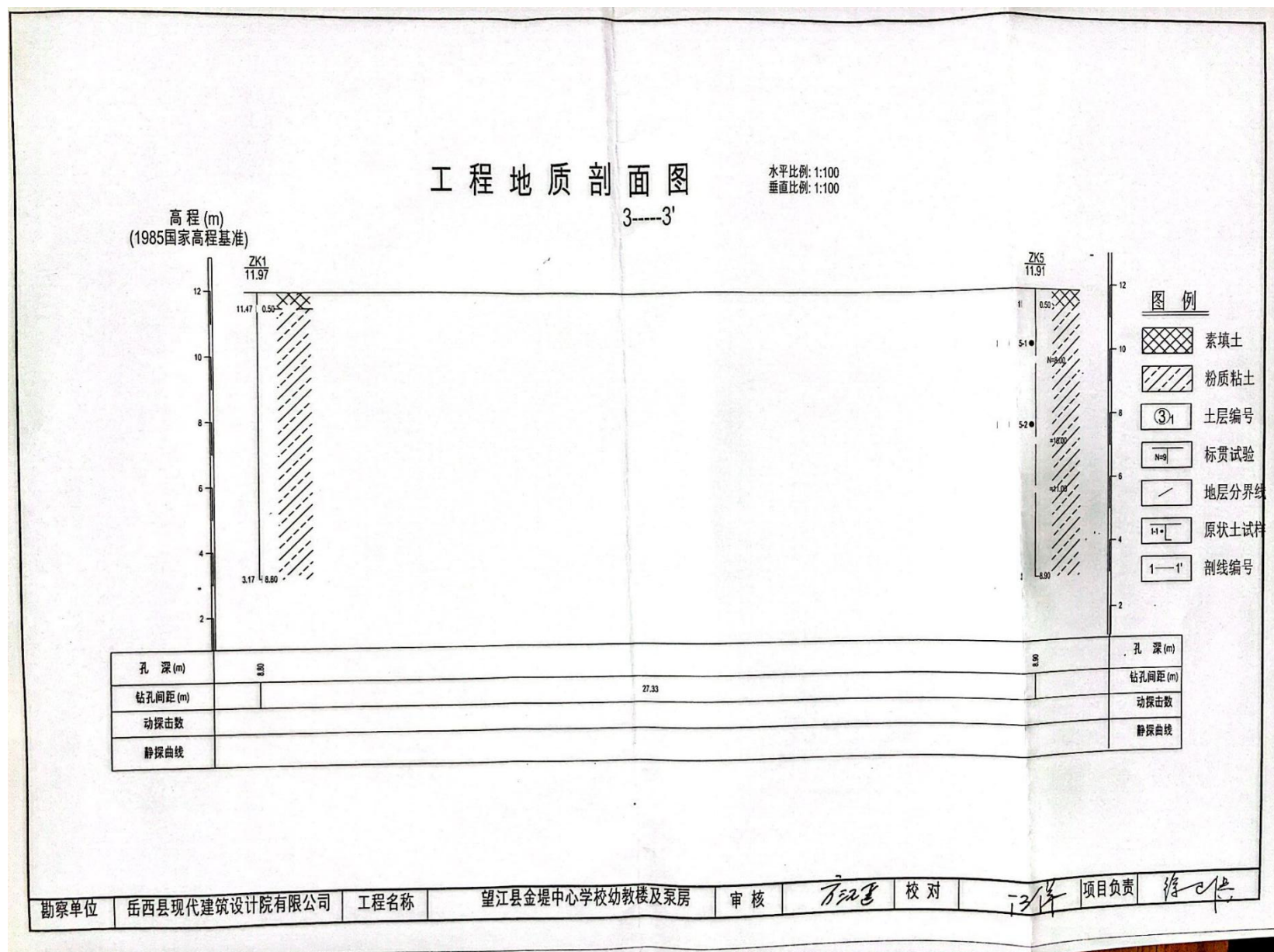
图 3-4 3-3'工程地质剖面图
