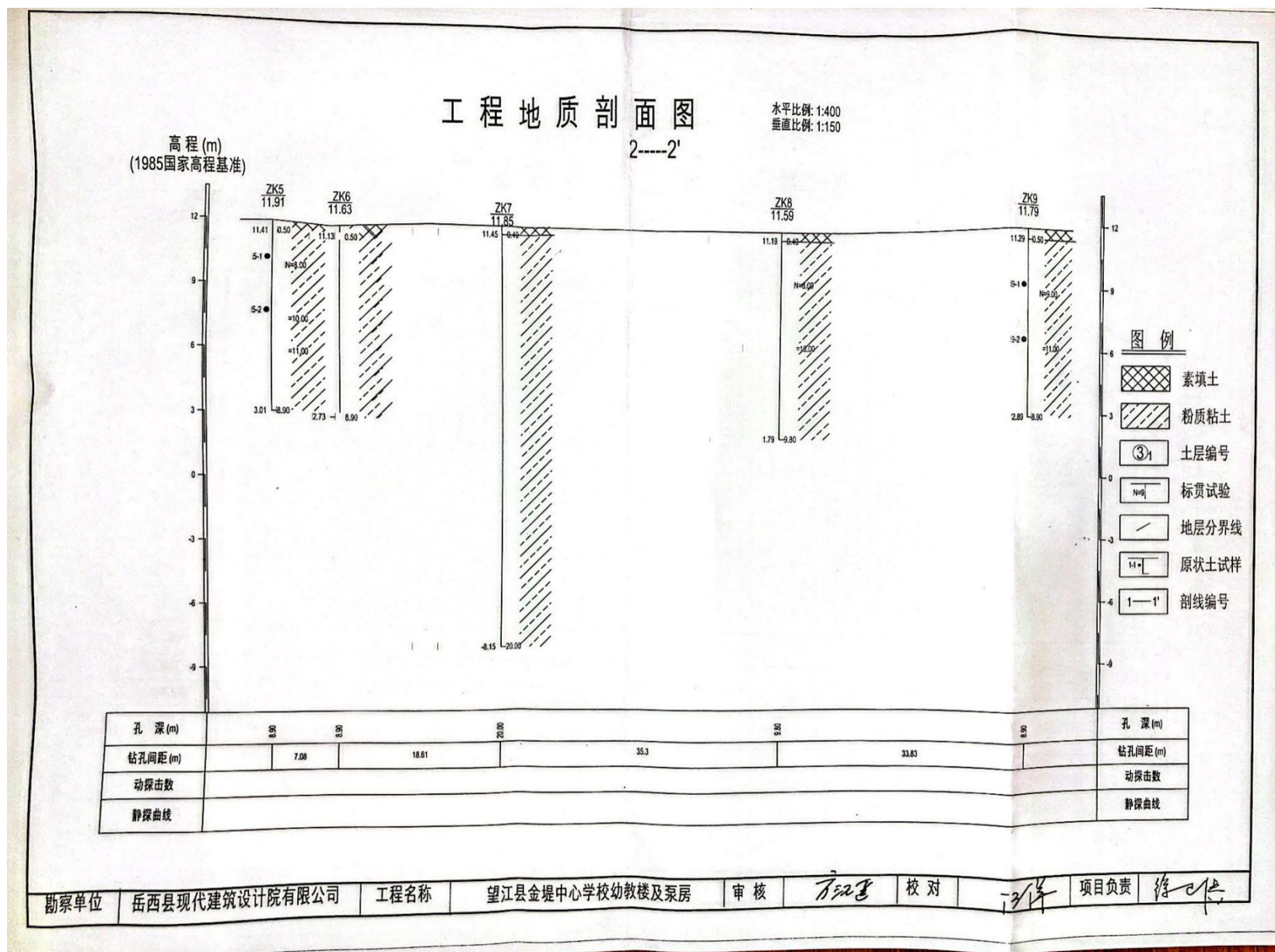
图 3-3 2-2'工程地质剖面图
