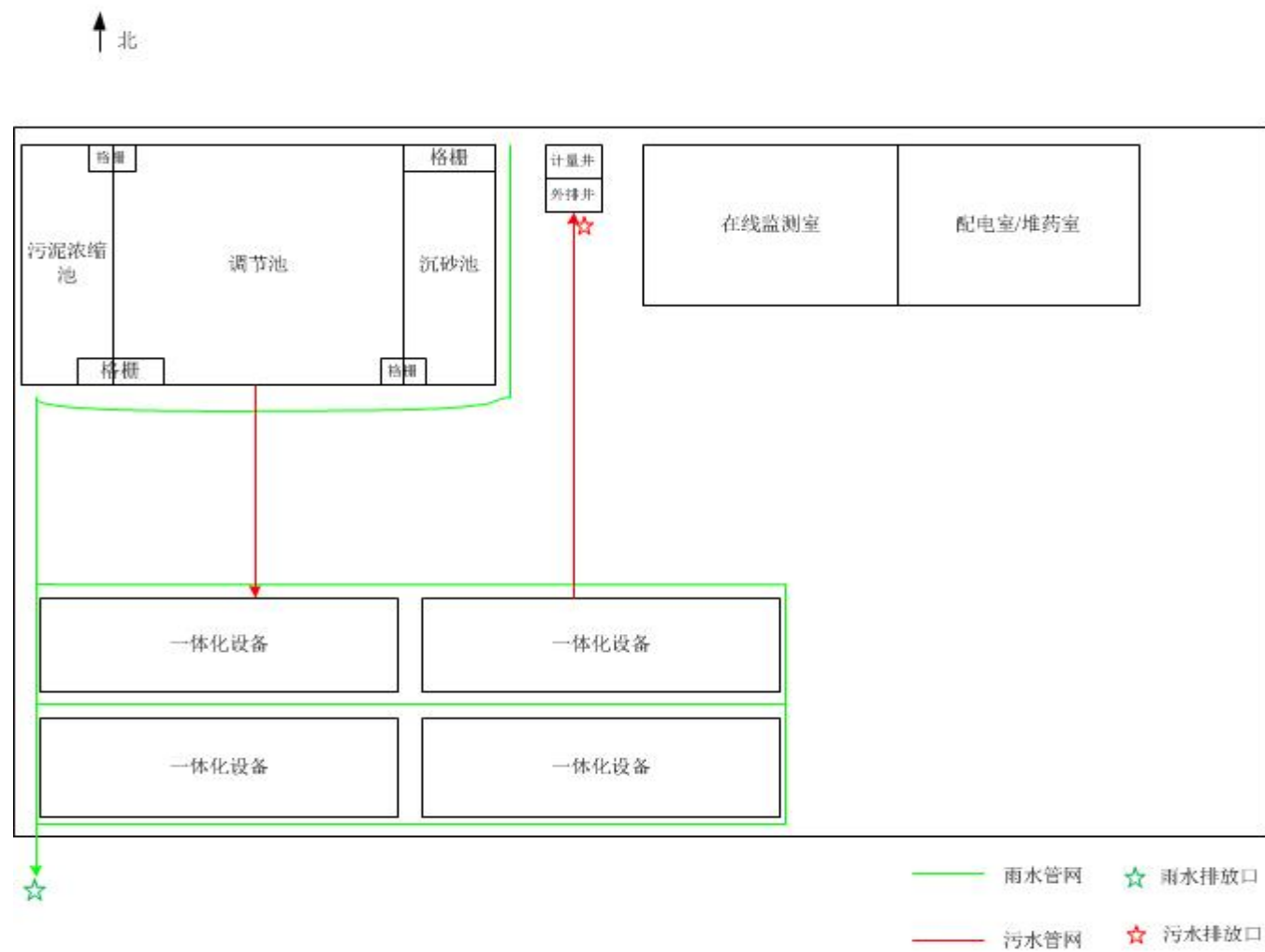
附图二：本项目平面布置图
