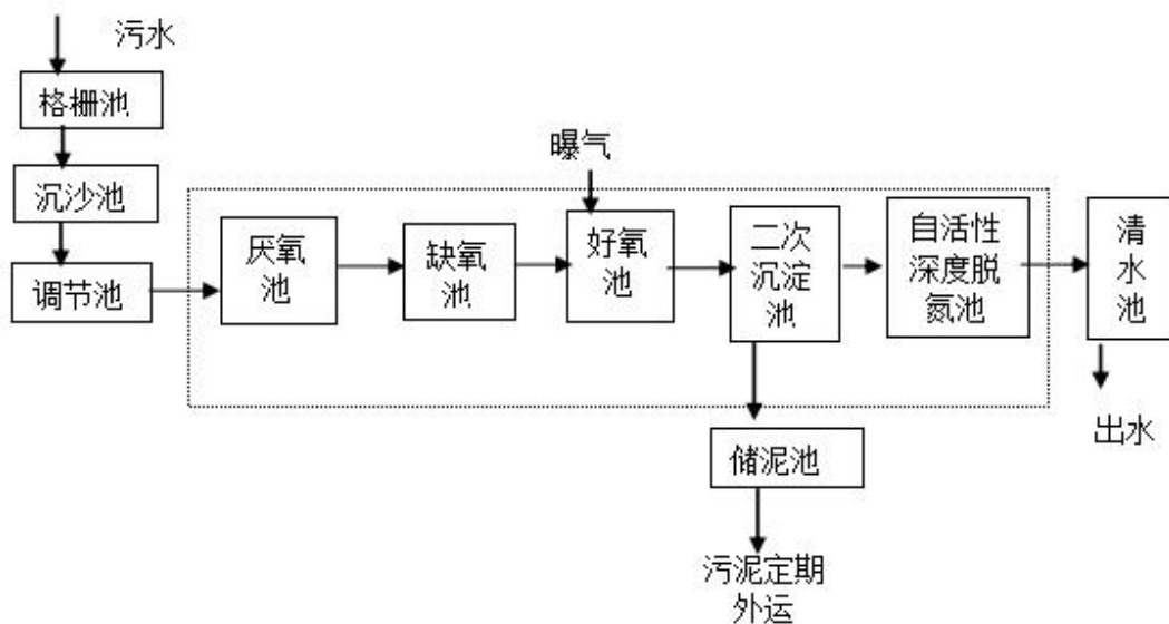
图2-2 环评设计污水处理工艺流程图
