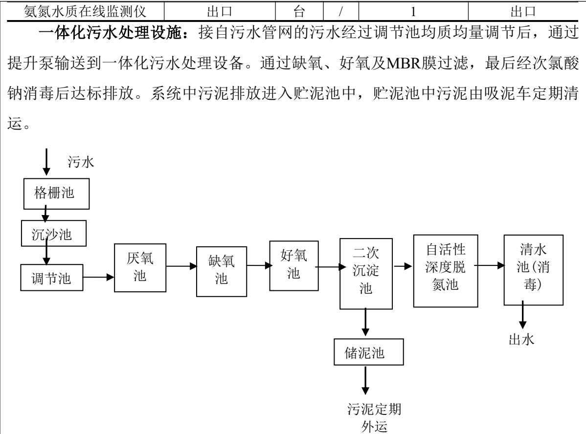
图2-1 污水处理设施工艺流程图
