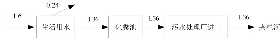
图2-1 项目水平衡图
