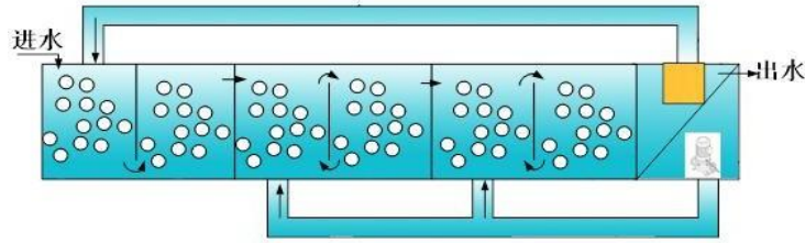
图 2-2 MBBR 除污染物原理示意图
