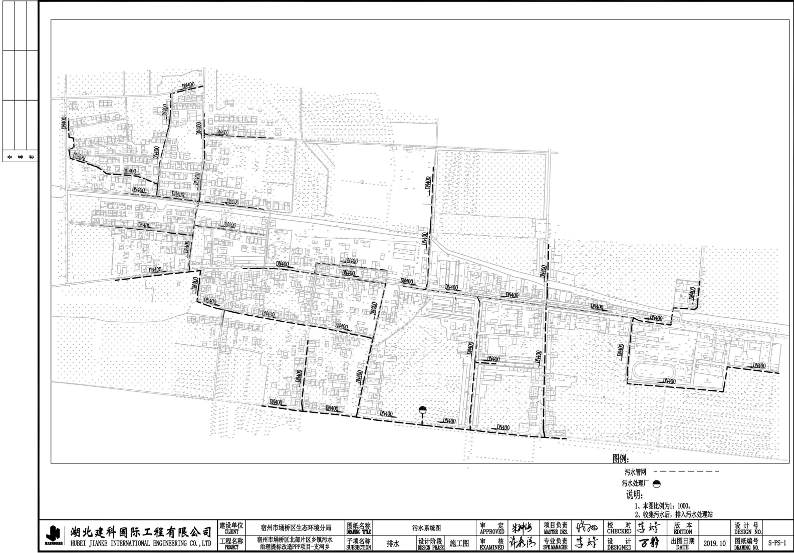
附图四 管网施工设计图
